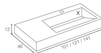
FRONTE CAIRO SOLID SURFACE - DERECHA
