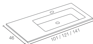
HERO SOLID SURFACE - DERECHA
