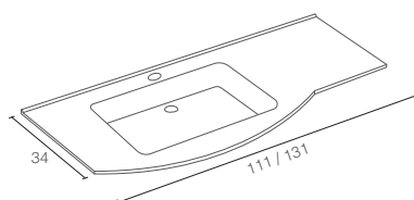
NEW PORT SOLID SURFACE - IZQUIERDA
