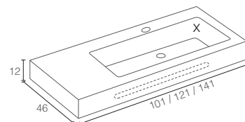
FRONTE HERO SOLID SURFACE - DERECHA
