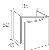
04 TRIPOLI - Puerta / Porte / Door
