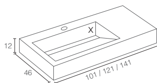
FRONTE CAIRO SOLID SURFACE - IZQUIERDA
