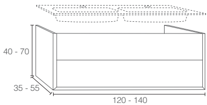
01 MONACO - Especial / Spécial / Special
