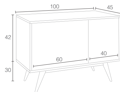
01 VINTAGE - Cajón, puerta - Tiroir, porte - Drawer, door
