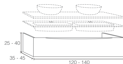
01 TRIPOLI - Especial / Spécial / Special
