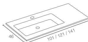
HERO SOLID SURFACE - IZQUIERDA
