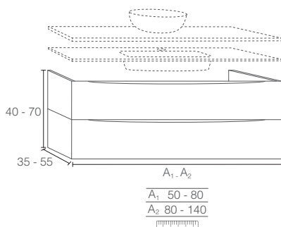
02 TRIPOLI - Especial / Spécial / Special
