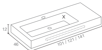
FRONTE HERO SOLID SURFACE - IZQUIERDA
